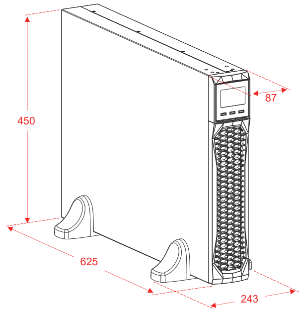
Installazione TOWER (dimensioni in mm)
