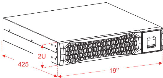
Installazione RACK
