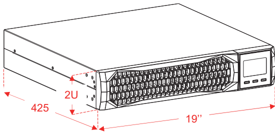
Installazione RACK
