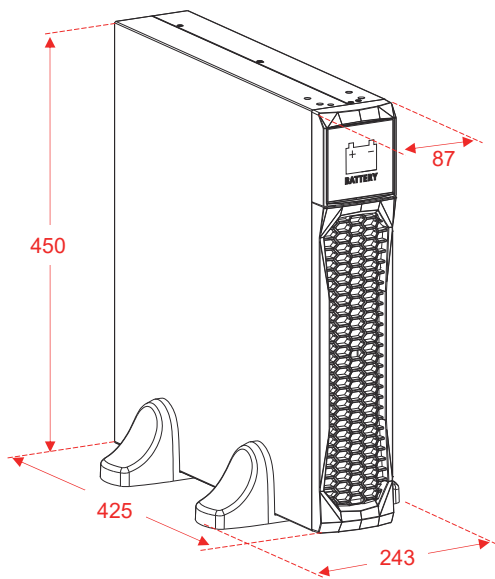
Installazione TOWER (dimensioni in mm)
