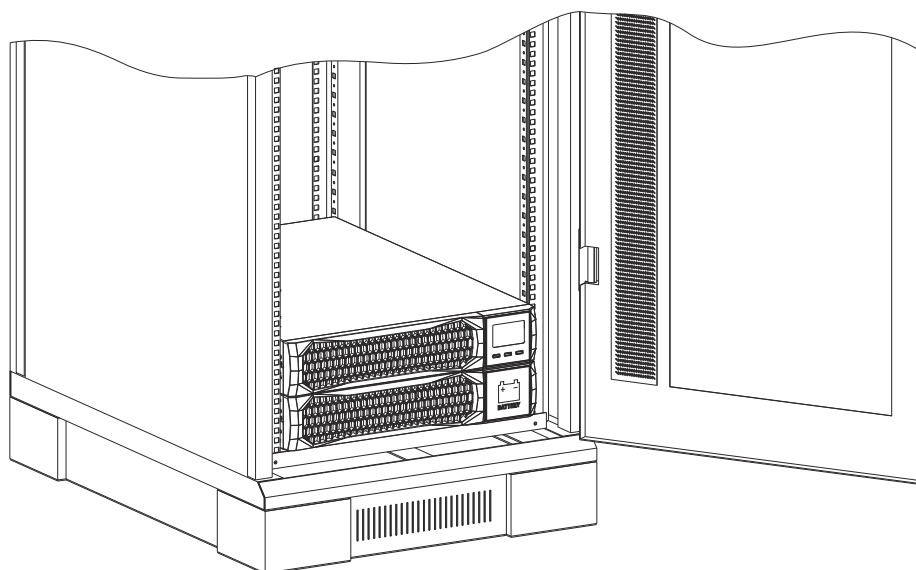
Esempio di UPS e BATTERY CABINET (opzionale) installati in posizione rack
