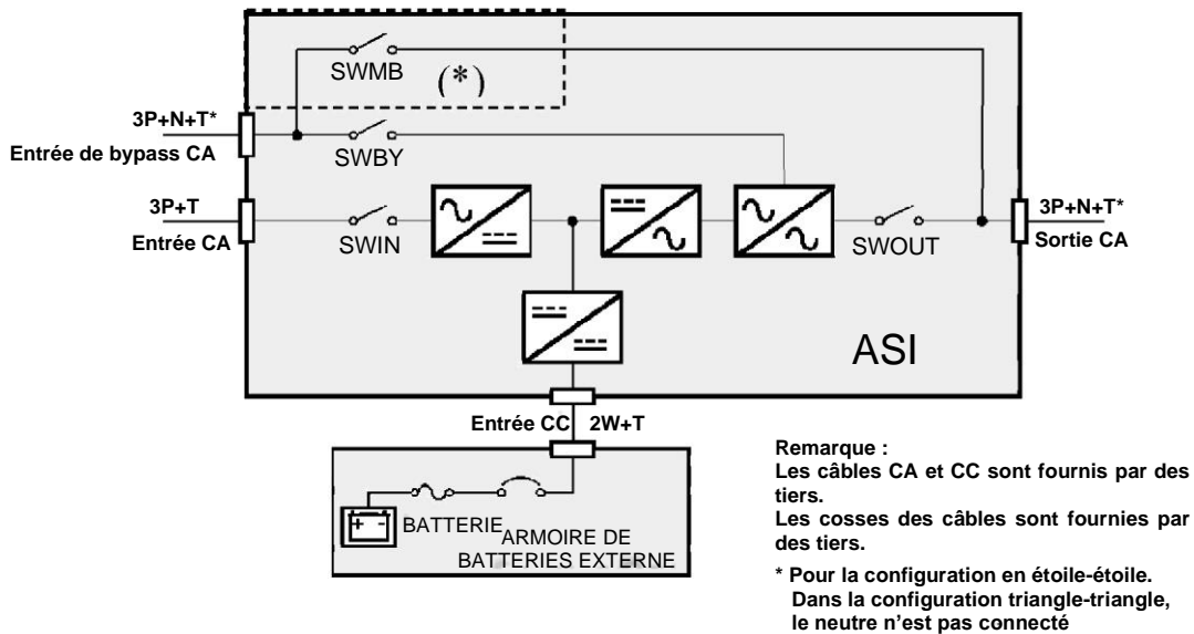
Schéma : Deux appareils d'entrée
