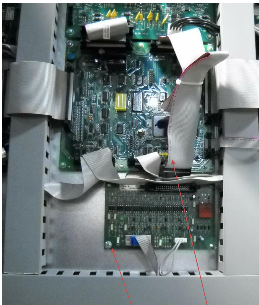
Câble déconnecté Carte de commande de la mise en parallèle
