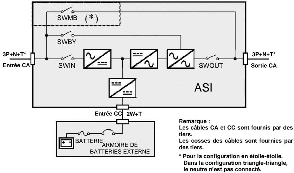
Schéma : Un appareil d'entrée
