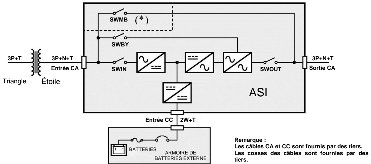
Schéma : Circuit d'alimentation unique sans neutre depuis la source
