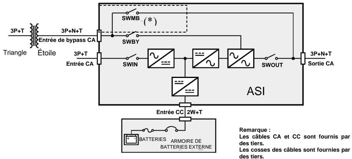
Schéma : Alimentation secteur et bypass séparé sans neutre depuis la source
